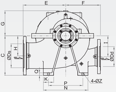
球墨铸铁法兰尺寸25bar（JIS 20K）
