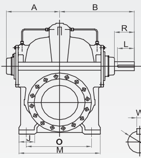
铸铁法兰尺寸16bar（JIS 16K）
